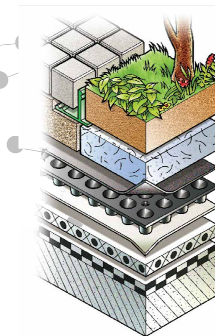
Διαστρωμάτωση υλικών συστήματος "πράσινου δώματος" EshaOxygen
